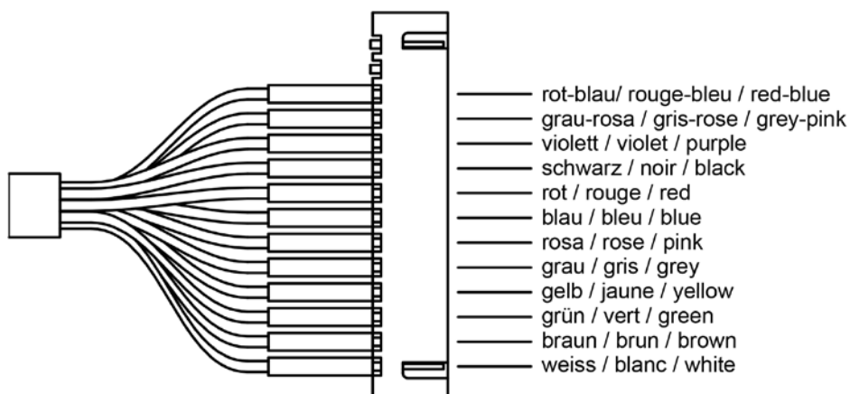
11104 - Kabeladapter HZ-lock VB zu MINT ELK Massbild
